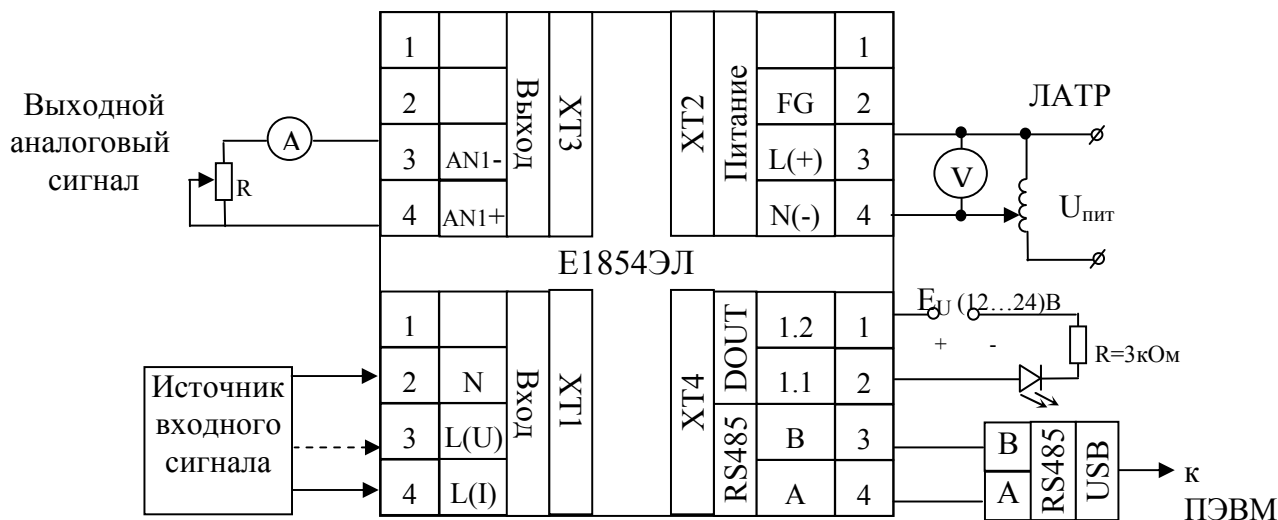
Рисунок В.1 – Схема подключения преобразователя E1856ЭЛ
